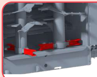
Einklappbare Wurfschaufeln auf Verschleißring montiert für bessere Krümelung.
