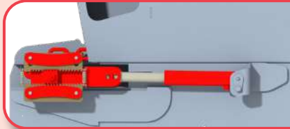
Hydraulischer Transportbodenspanner mit automatischer Spannsicherung
