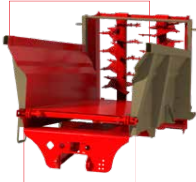
Caja abocardada de una sola pieza con chapas laterales de una sola pieza para facilitar la extracción del producto.
