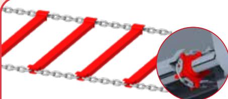
Buisvormige latten gelast aan scheepvaartkettingen 14 (om materiaalopslag te voorkomen) + mechanisch gelaste tandwielen.
